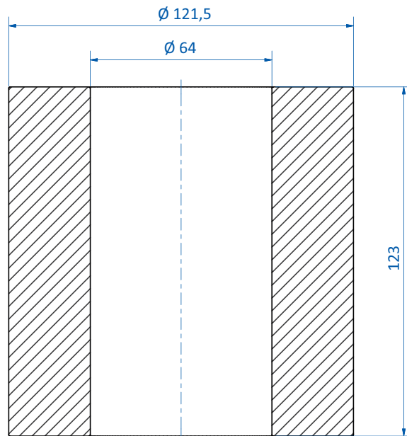
FC 40F-Kartusche
