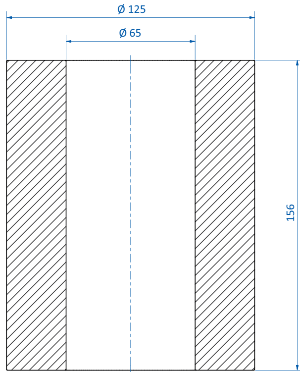
FC 50F-Kartusche
